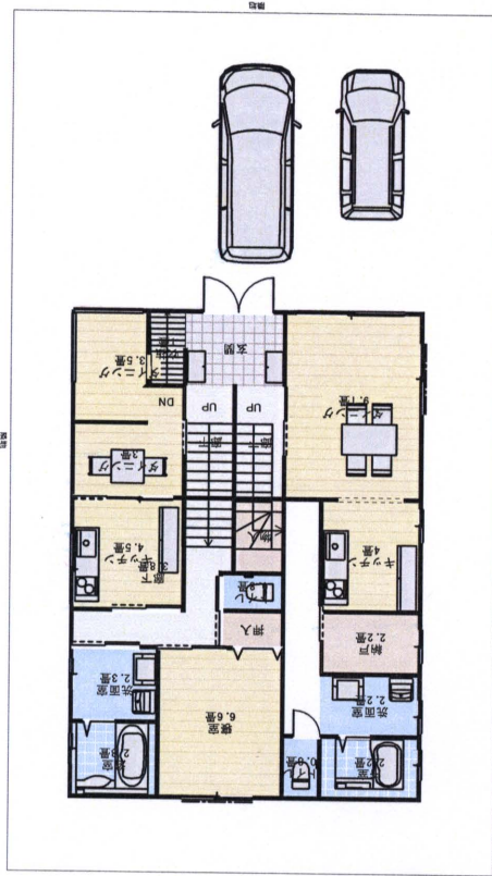
1階縮尺1/200
